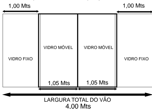
Porta de 2 folhas móveis e 2 folhas fixas.
